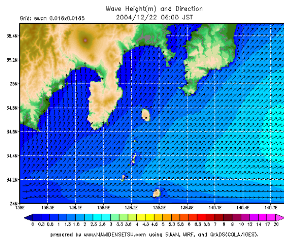
図-1 波浪予測計算の例(上段:領域R00;下段:領域R02)
