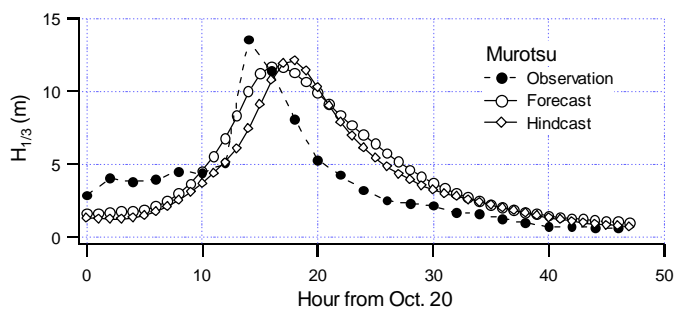
図 - 7 室津における波高観測値および予測値、追算値の比較
