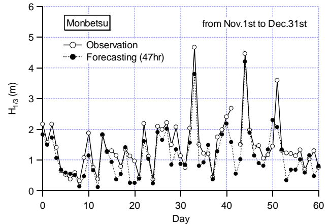
図-2 紋別における波高の観測値および予測値の時系列
